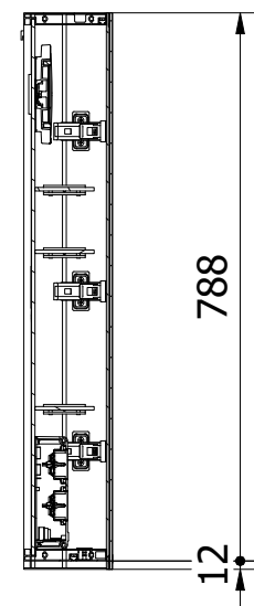
B-B ( 1 : 12 )
