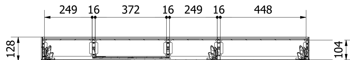
A-A ( 1 : 12 )
